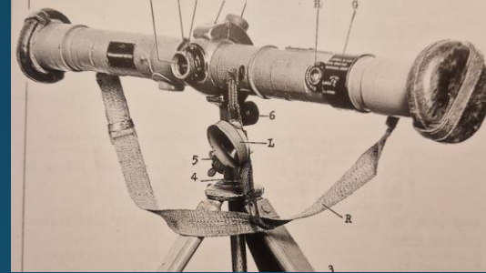
Koinsidenssietäisyysmittari
